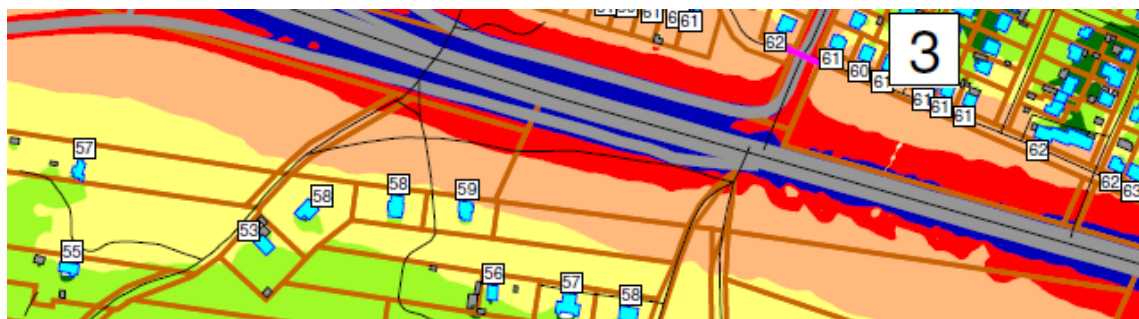
Joonis 3 Väljavõte Tallinna ringtee km 30,1 – 34,5 Kanama - Valingu põhiprojektist: liiklusmüra modelleerimine”, 2017 ehitusjärgne olukord müratõkkeseinteta kaardist päevasel ajal.
