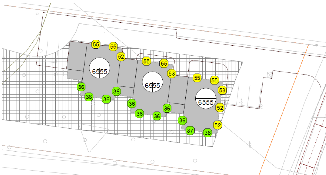
Joonis 15. Hoonete välispiiretele mõjuvad müratasemed, 2040.a. liiklussagedused, öö LpA,eq (väljavõte Akukon Eesti OÜ 22.08.2023 koostatud uuringust “Aila küla Reinu kinnistu ja lähiala detailplaneeringule liiklusringist põhjustatud müratasemete hindamine”).
