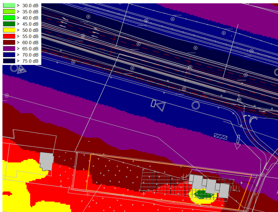
Joonis 12. Autoliiklusest põhjustatud müratasemed päevasel ajavahemikul (7-23), Ld (väljavõte Akukon Eesti OÜ 22.08.2023 koostatud uuringust “Aila küla Reinu kinnistu ja lähiala detailplaneeringule liiklusrast põhjustatud müratasemete hindamine”).
