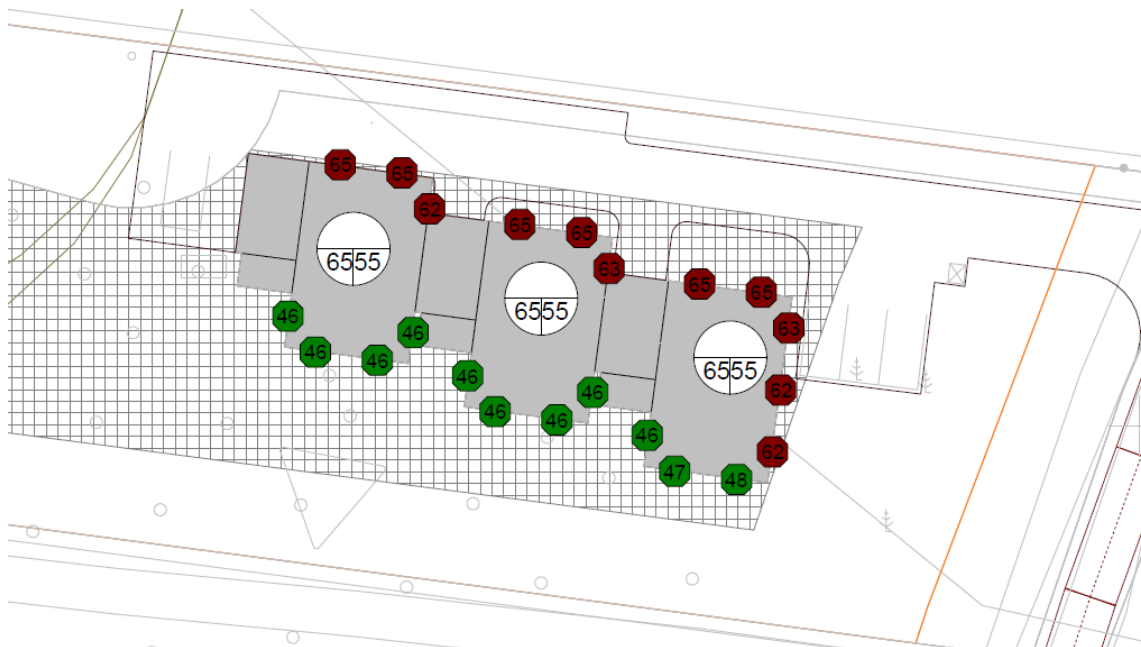
Joonis 14. Hoonete välispiiretele mõjuvad müratasemed, 2040.a. liiklussagedused, päev LpA,eq (väljavõte Akukon Eesti OÜ 22.08.2023 koostatud uuringust “Aila küla Reinu kinnistu ja lähiala detailplaneeringule liiklusringist põhjustatud müratasemete hindamine”).
